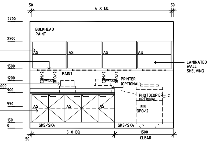
ELEVATION 2
