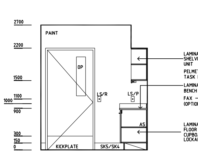
ELEVATION 1
